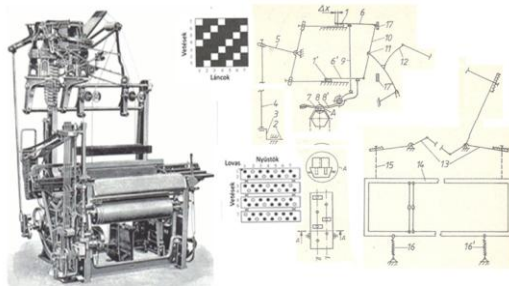
5. ábra: Hattersley kétütemű nyüstösgép vázlatja
