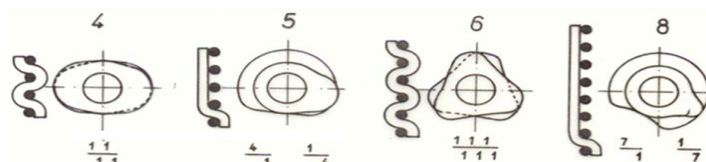
3. Ábra: Különböző raportú, különböző kötést megvalósító bütyökpárok
