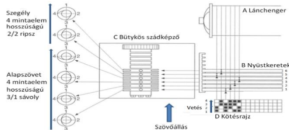
4. ábra: Adott kötést megvalósító bütykök összeszerelése
