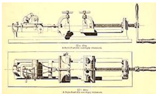
8. ábra: A Rejtő-Králik szakító-gép felülnézeteben "A papíros tartóssága" című könyvből [5]
